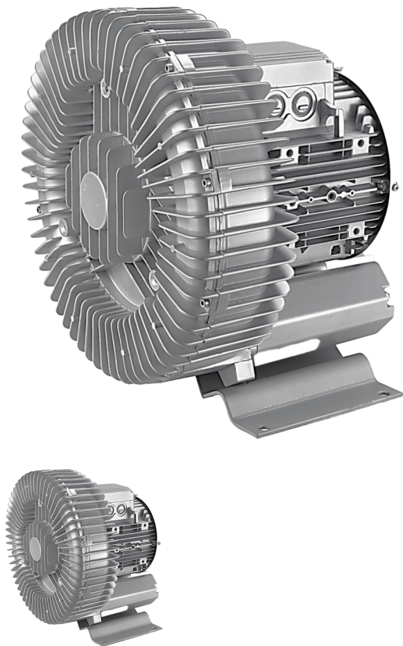
Légfűvő 720T 5,5kW/400V, 320m3/h 500mbar
