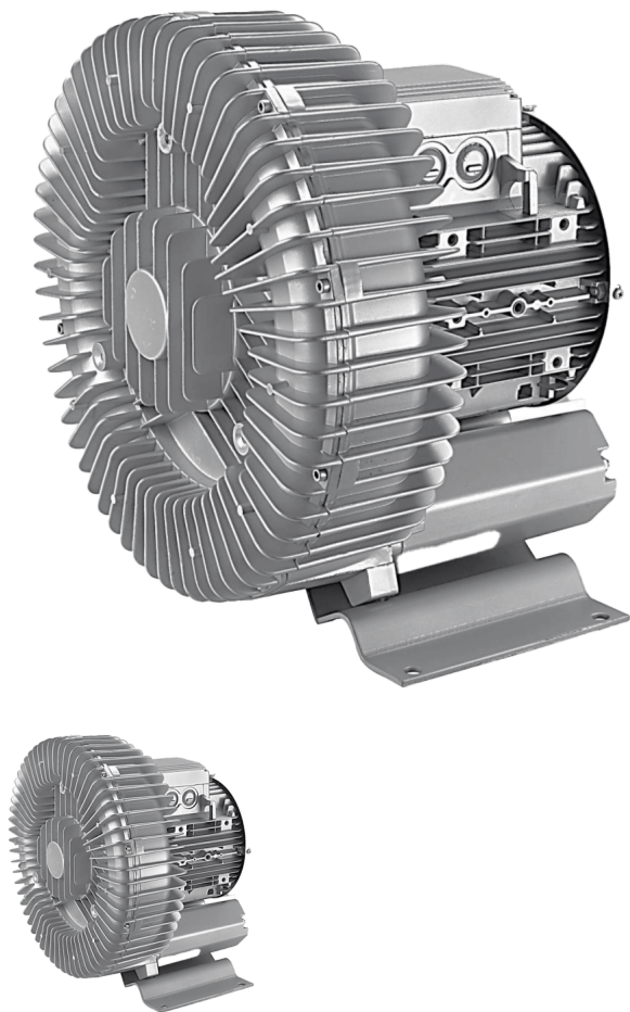
Légfúvó 430T 1,3kW/400V, 180m3/h 180mbar
