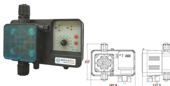
Microdos ME1-CA 2l/h - 12bar
