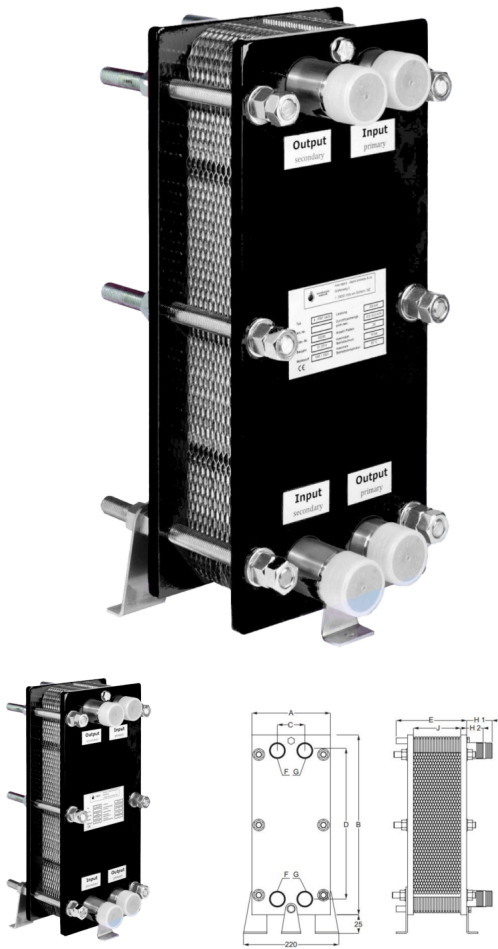
Lemezes hűtőcserél? Power 13M-PWT 1327M-VA - 500 kW - 70°C
